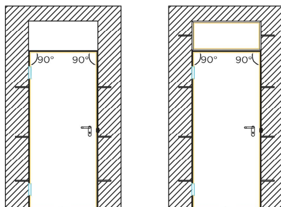
PLACEMENT DE LA PORTE DANS SA RESERVATION
