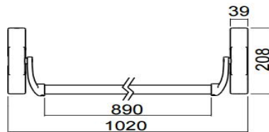
Modele Anti-panique 1970 (standard : BA1)
