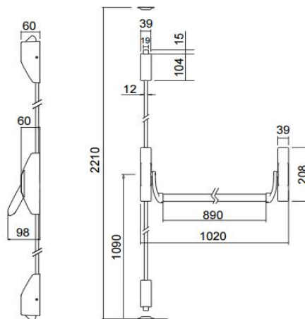
Modele Anti-panique 1930 (standard : BA8)
