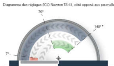
Montage Standard avec Glissière K, Côté opposé paumelles.
