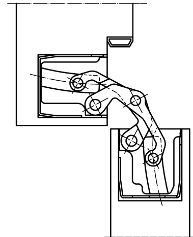
bloc-porte 90°
