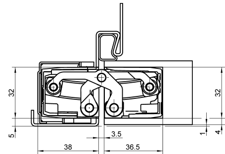
huisserie métallique
