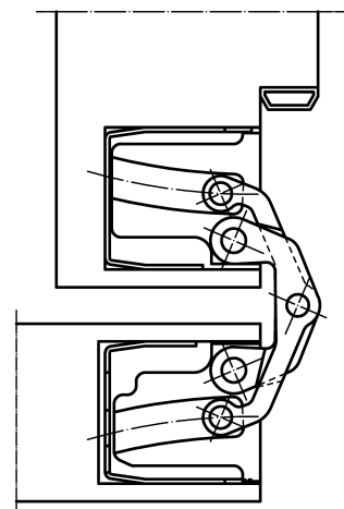
bloc-porte 180°
