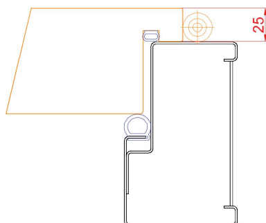
Retour contre dormant, épaisseur 25mm
