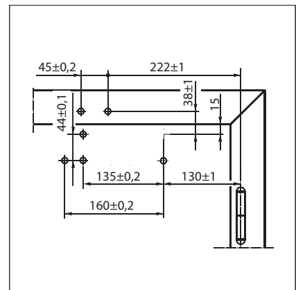
Cotes de montage porte de droite
