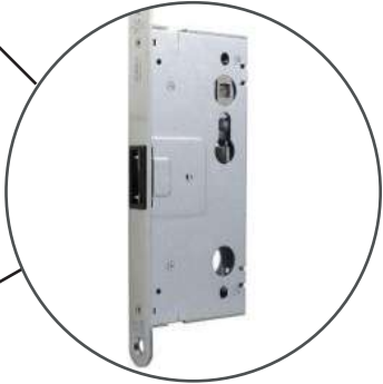
Crémone Pompier encastrée
